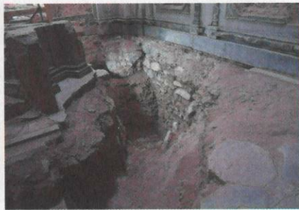
Fig. 7. Vista d'una de les rases que gairebé assolia els 3 m de fondària.
