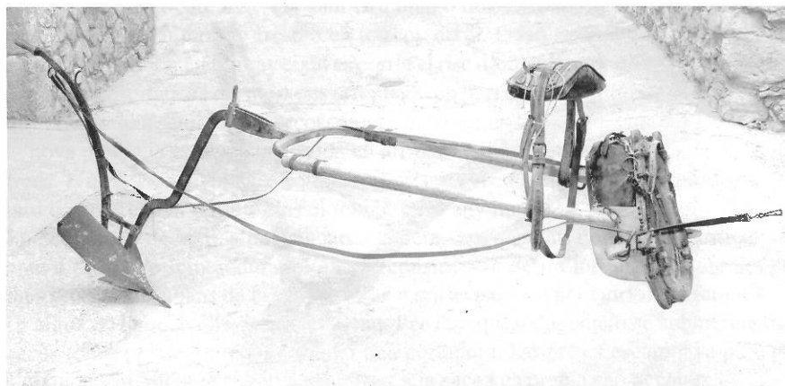
Muntatge fet amb la pollegana i els arreus en disposició de llaurar. Foto de Carles Segarra
