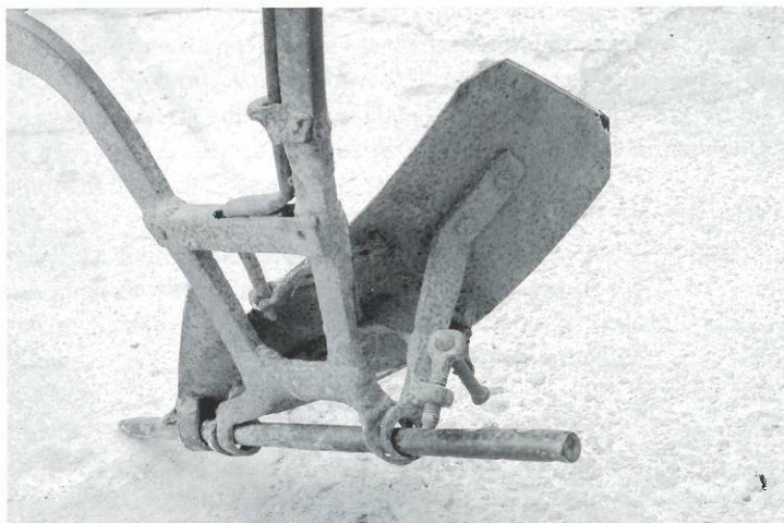
Detall del mecanisme de fixació de la rella i de gir de la pala.
