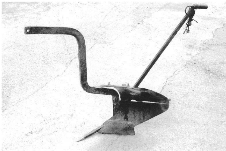
Pollegana amb el mecanisme de pala giratòria per dalt.
