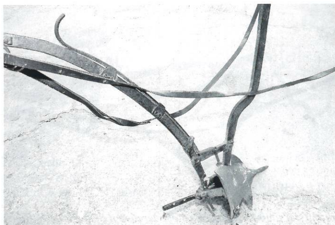
Detall de la pollegana amb la pala giratòria, aquesta s'havia de girar per baix de la rella. Foto de Carles Segarra.
