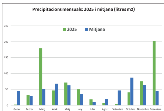
Gràfic 1: Comparativa entre l'any 2025 i la mitjana climàtica (1986-2025)
