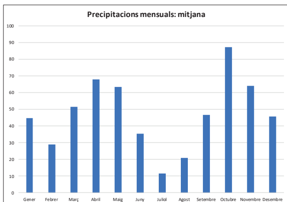
Gràfic 9: Mitjanes de les precipitacions mensuals
