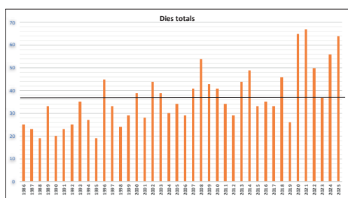
Gràfic 3: Dies de pluja anual
