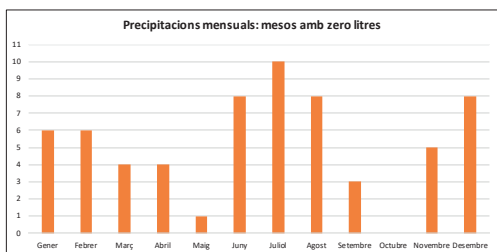
Gràfic 10: Nombre de mesos sense cap precipitació
