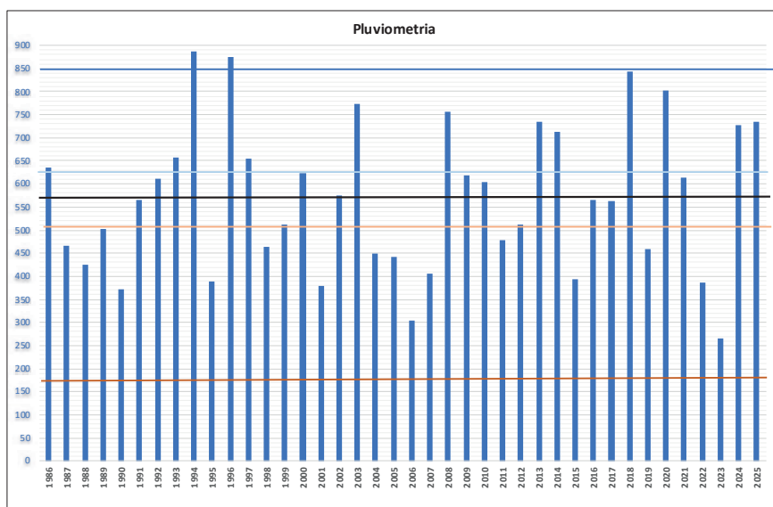
Gràfic 2: Precipitació anual. Tipus d'anys respecte de la mitjana climàtica segons la classificació del Meteocat:
